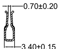
剖面 B-B
