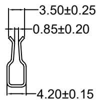
剖面 A-A
