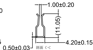
剖面 C-C
