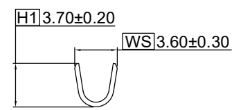
截面B-B
